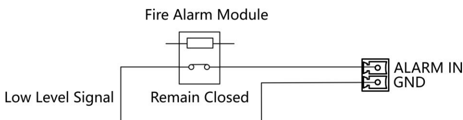
Рисунок 5-9 Оставить закрытым
